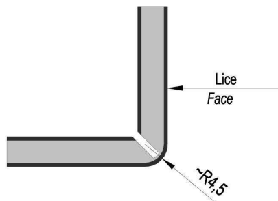
Izrada žljeba za savijanje pod uglom 90° V- Shaped Groove for 90° folding
