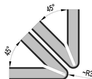
Izrada žljeba za savijanje pod uglom 45° V- Shaped Groove for 45° folding
