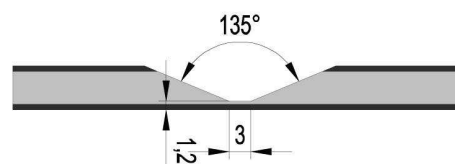
Izrada žljeba za savijanje pod uglom 45° V- Shaped Groove for 45° folding
