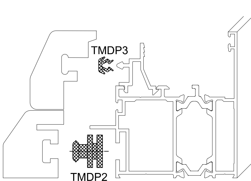
Nosač drveta Wood holder Держатель дерева
