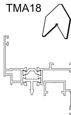
Spojница u peru Thorn clip Клип в шипе
