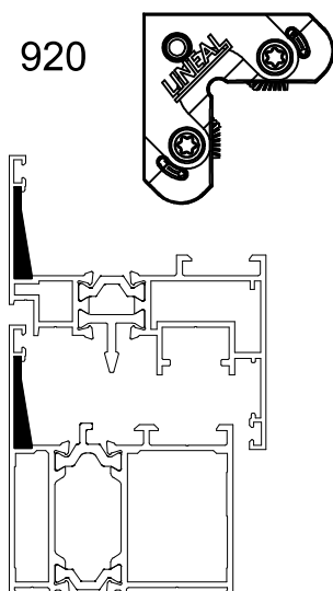
Spojница u peru Thorn clip Клип в шипе
