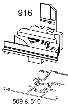
Čep profila veze dvokrillnog prozora Double casement connection profile bung Затычка соединительного профиля двойной створки
