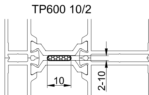
Penasti profil na spoju Joint foam profile Профиль пены на суставе
