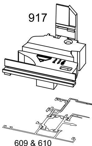
Čep profila veze dvokrillnog prozora Double casement connection profile bung Затычка соединительного профиля двойной створки
